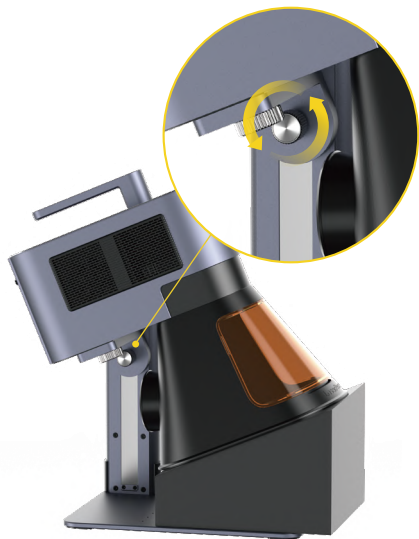
Drehvorrichtung
